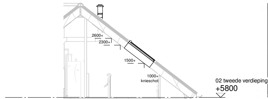
Doorsnede schaal 1:100
