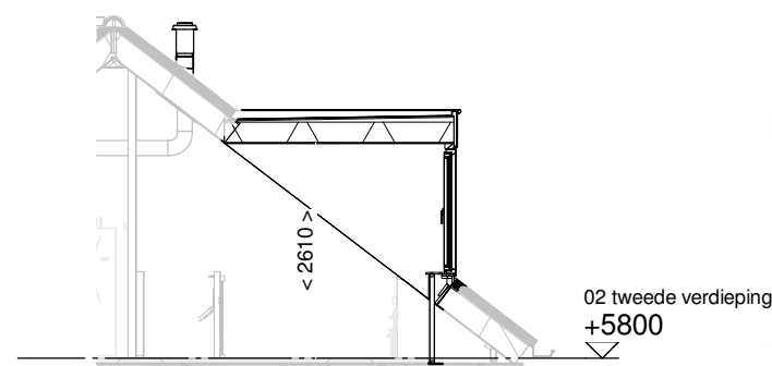
Doorsnede schaal 1:100
