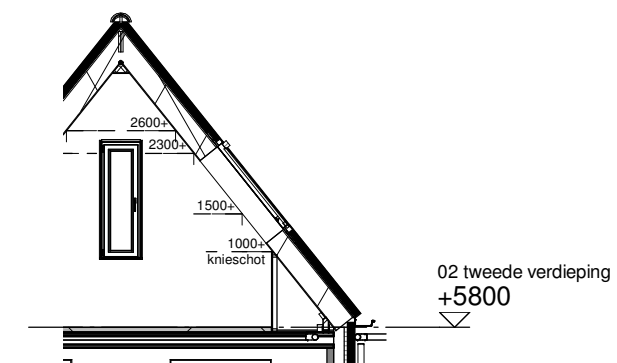
Doorsnede schaal 1:100
