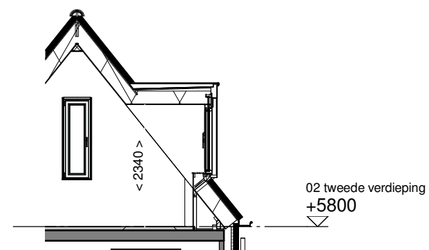
Doorsnede schaal 1:100
