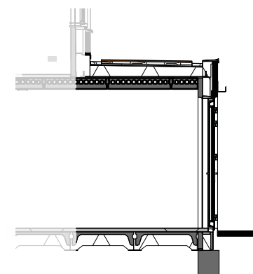
Doorsnede schaal 1:100
