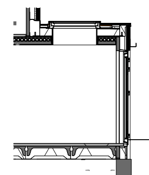
Doorsnede schaal 1:100
