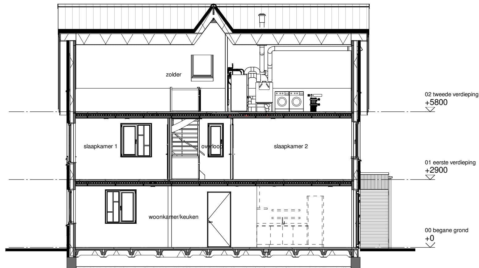
Doorsnede A
