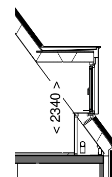
Doorsnede schaal 1:100
