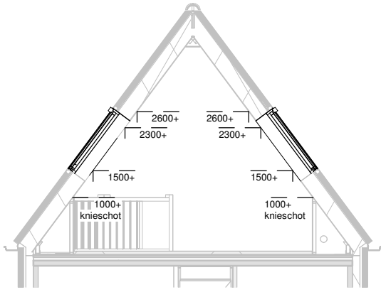
Doorsnede schaal 1:100
