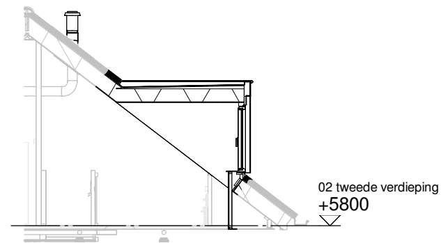
Achtergevel schaal 1:100
