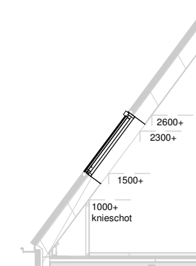
Doorsnede schaal 1:100
