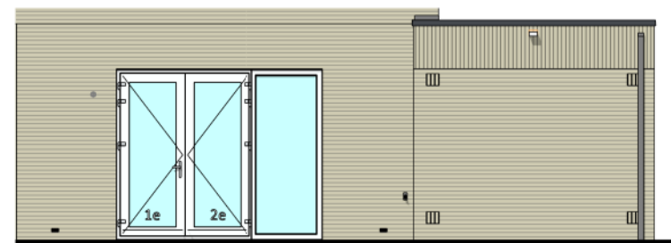
Achtergevel schaal 1:100
