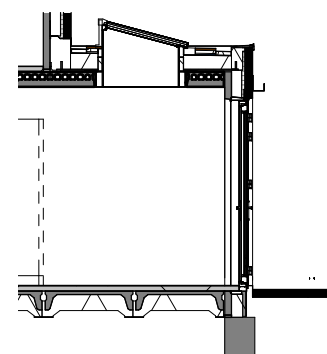
Doorsnede schaal 1:100
