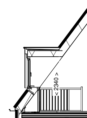
Doorsnede schaal 1:100
