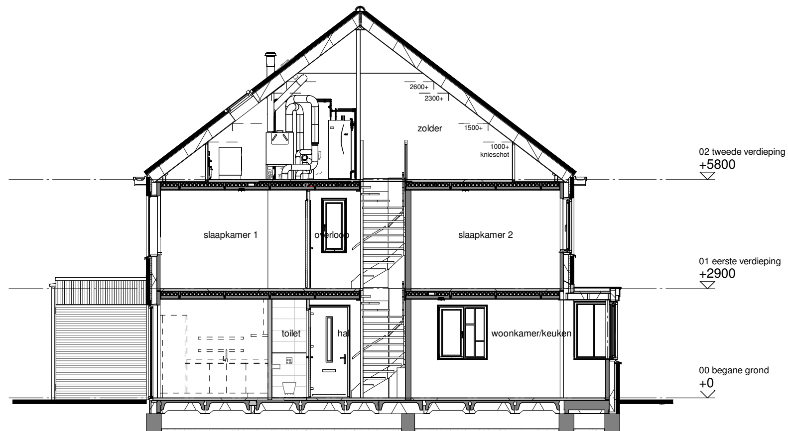
Doorsnede A
