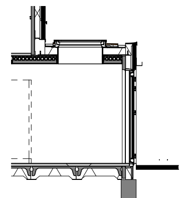
Doorsnede schaal 1:100
