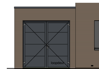
Voorgevel schaal 1:100
