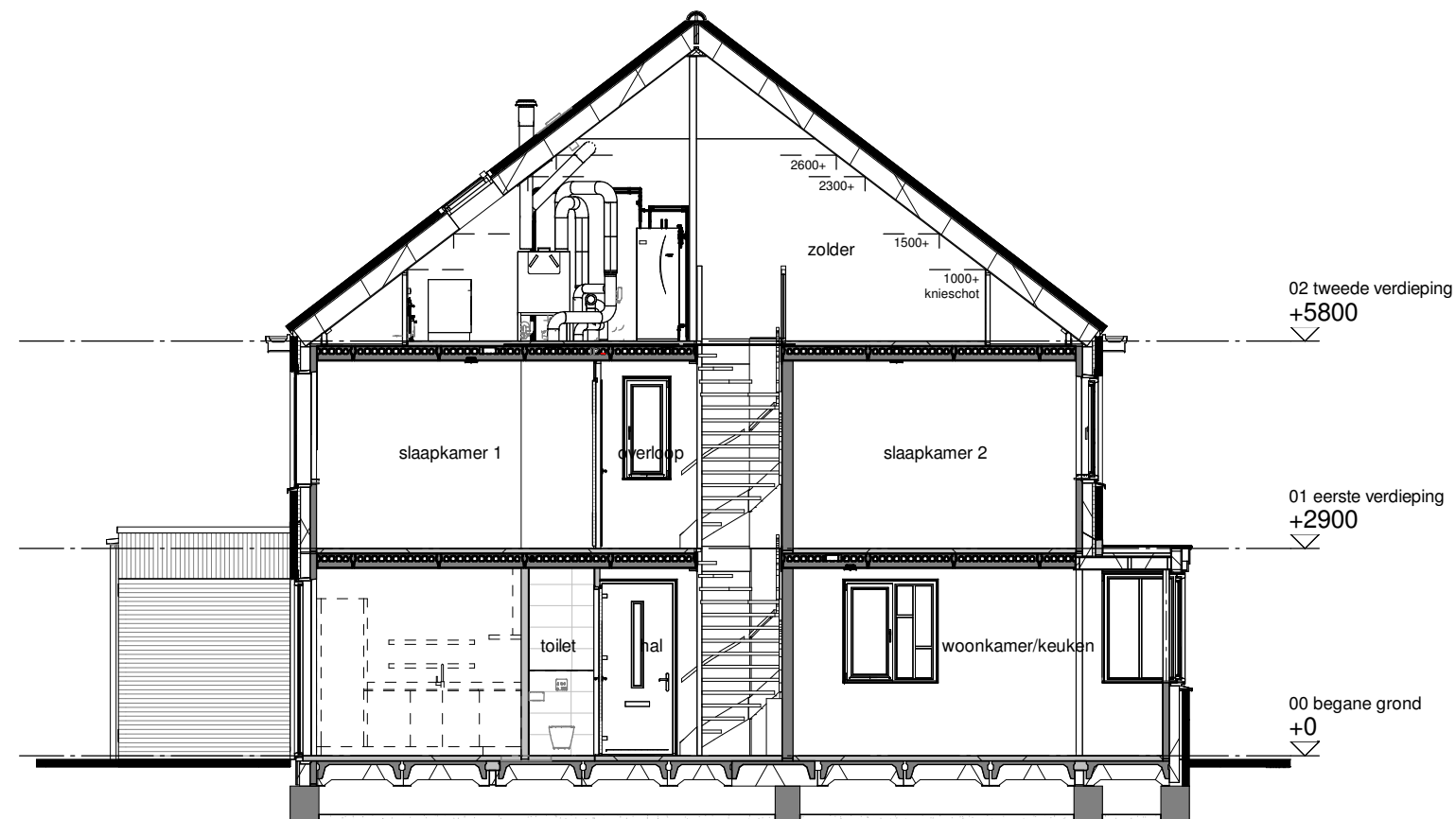
Doorsnede A
