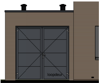
Voorgevel schaal 1:100
