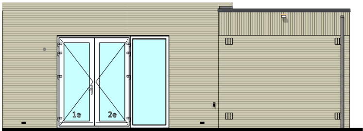
Achtergevel schaal 1:100
