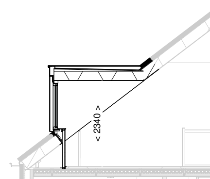
Doorsnede schaal 1:100
