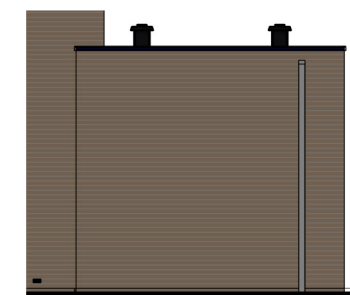
Achtergevel schaal 1:100
