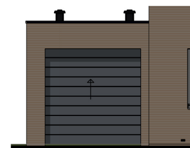
Voorgevel schaal 1:100
