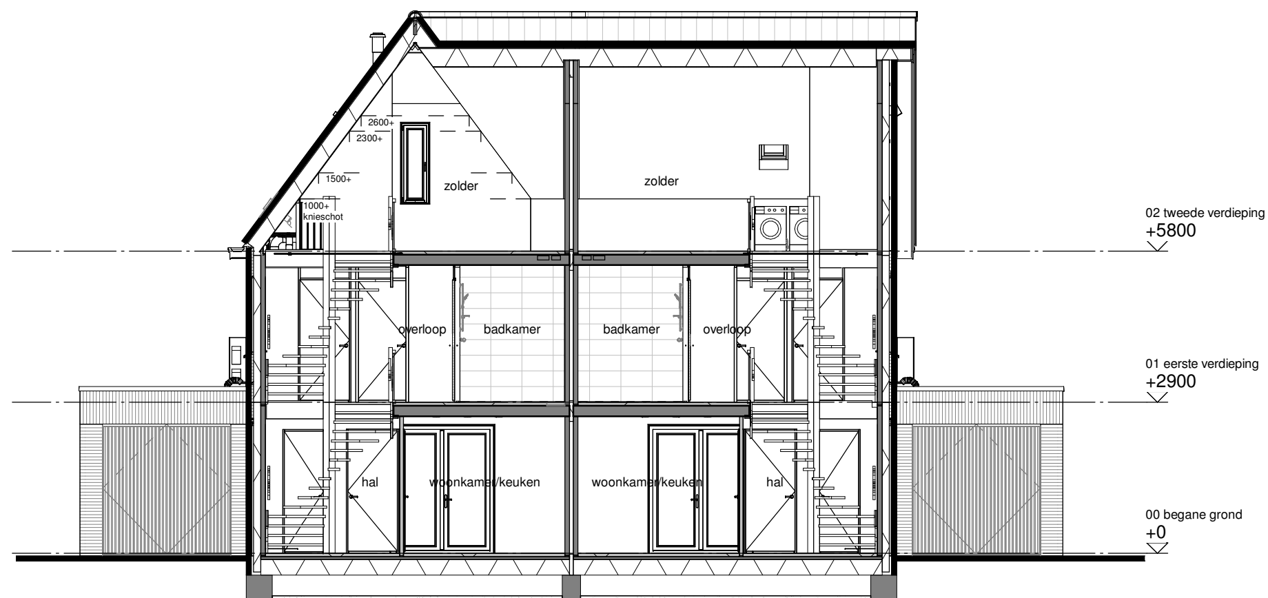
Doorsnede B
