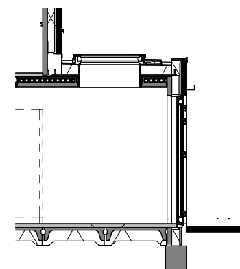
Doorsnede schaal 1:100
