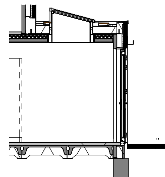
Doorsnede schaal 1:100
