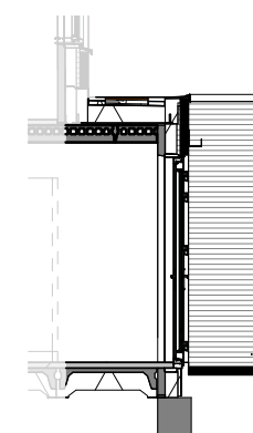
Doorsnede schaal 1:100
