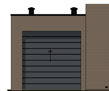
Voorgevel schaal 1:100
