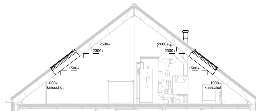
Doorsnede schaal 1:100
