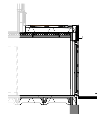
Doorsnede schaal 1:100
