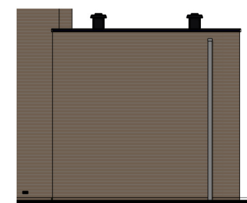
Achtergevel schaal 1:100
