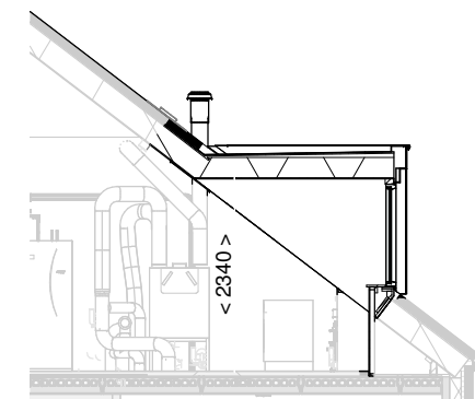
Doorsnede schaal 1:100
