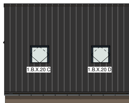
Vorgevel schaal 1:100
