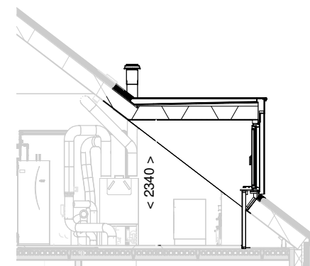
Doorsnede schaal 1:100
