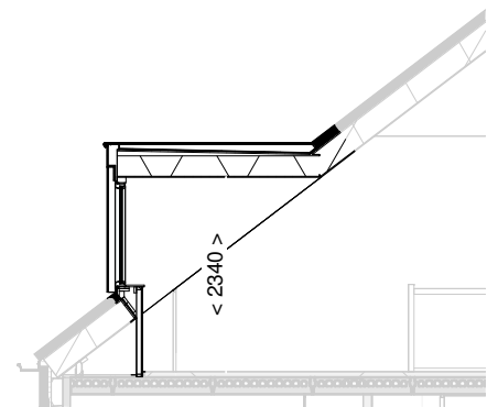
Doorsnede schaal 1:100
