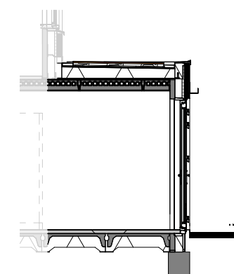
Doorsnede schaal 1:100
