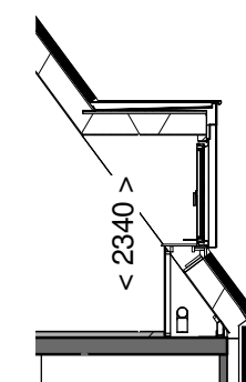
Doorsnede schaal 1:100
