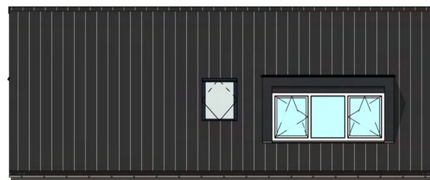
Linkerzijgevel schaal 1:100
