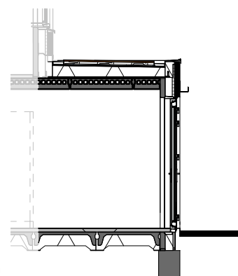
Doorsnede schaal 1:100
