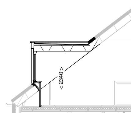
Doorsnede schaal 1:100
