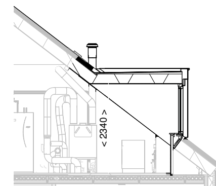
Doorsnede schaal 1:100
