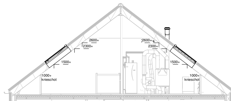
Doorsnede schaal 1:100
