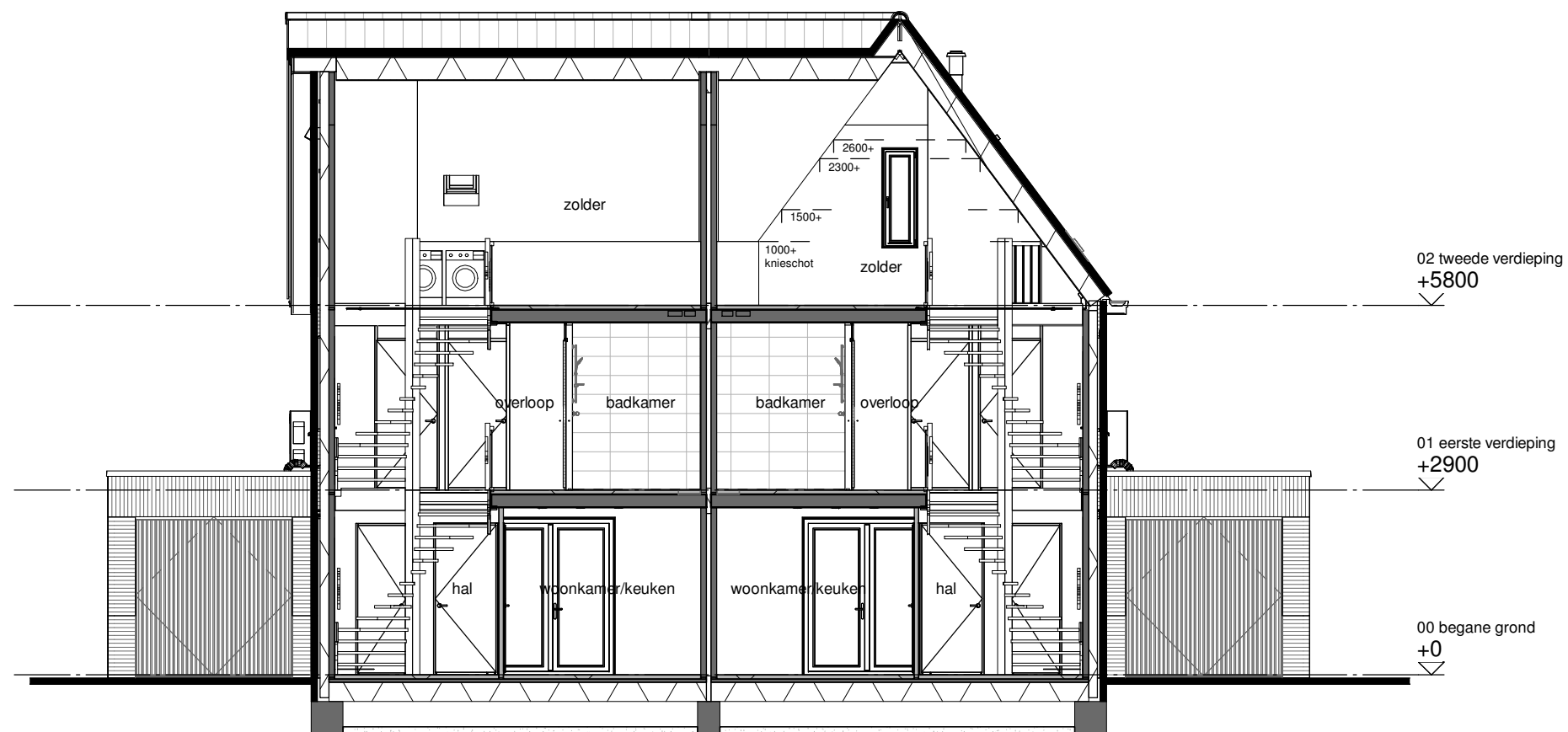
Doorsnede B
