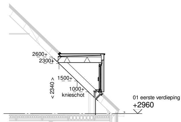
Doorsnede schaal 1:100
