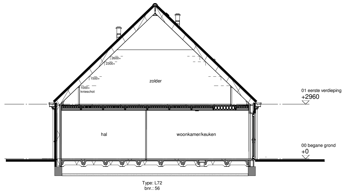
Doorsnede A
