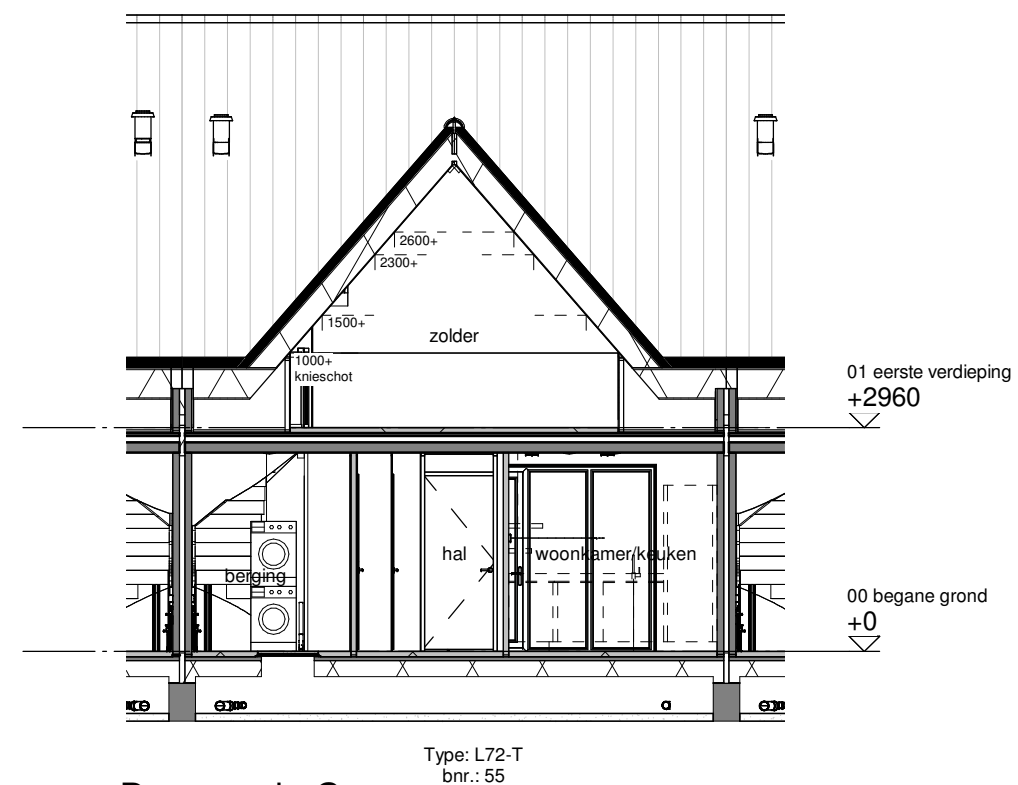
Doorsnede C
