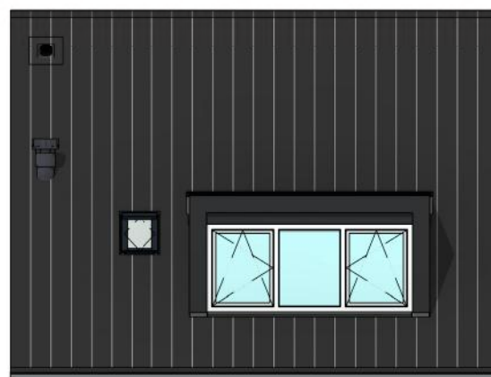
Achtergevel schaal 1:100
