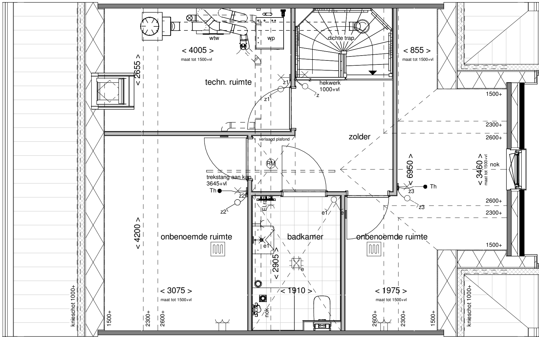
Eerste verdieping
