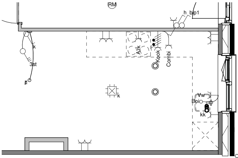
Begane grond
