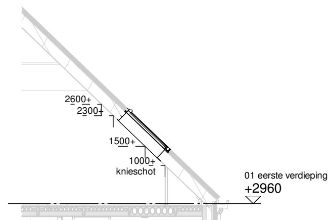
Doorsnede schaal 1:100
