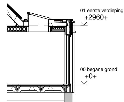
Doorsnede schaal 1:100
