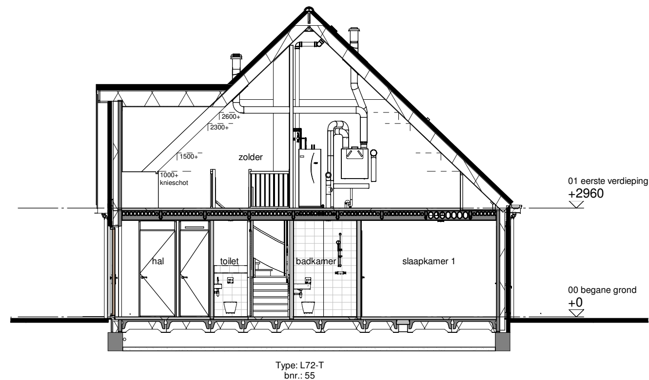
Doorsnede B
