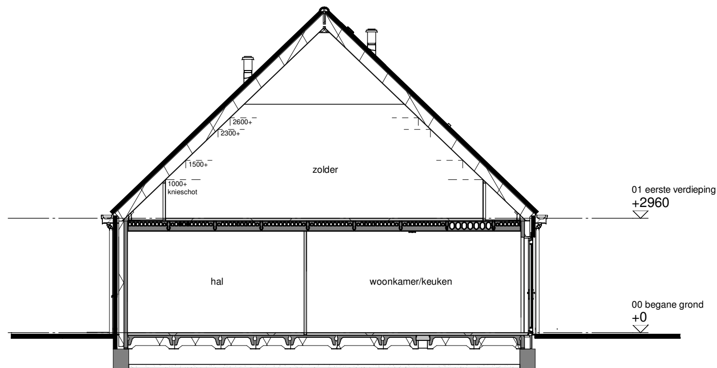
Doorsnede A
