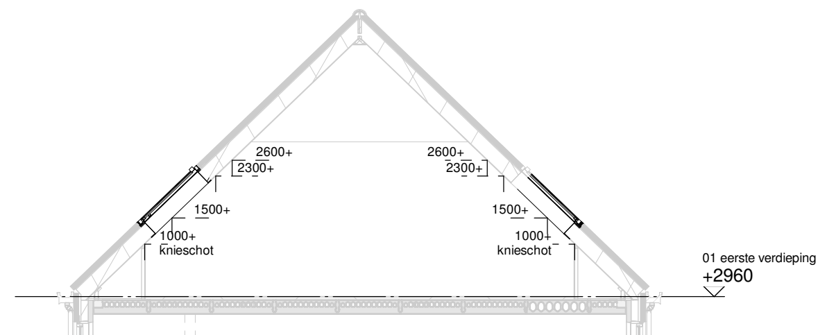
Doorsnede schaal 1:100
