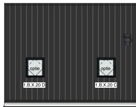
Voorgevel schaal 1:100
