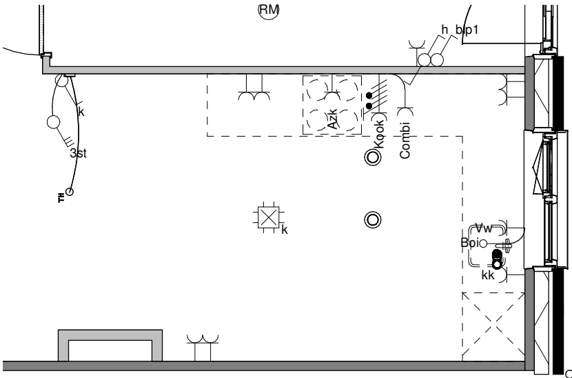
Begane grond
