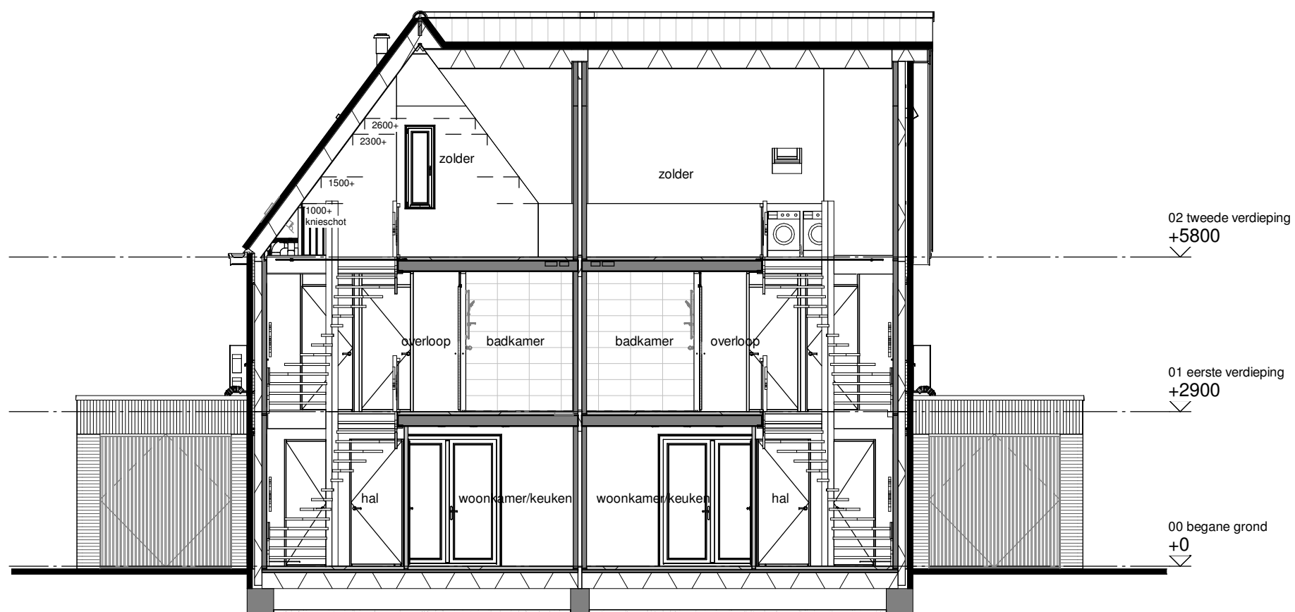
Doorsnede B
