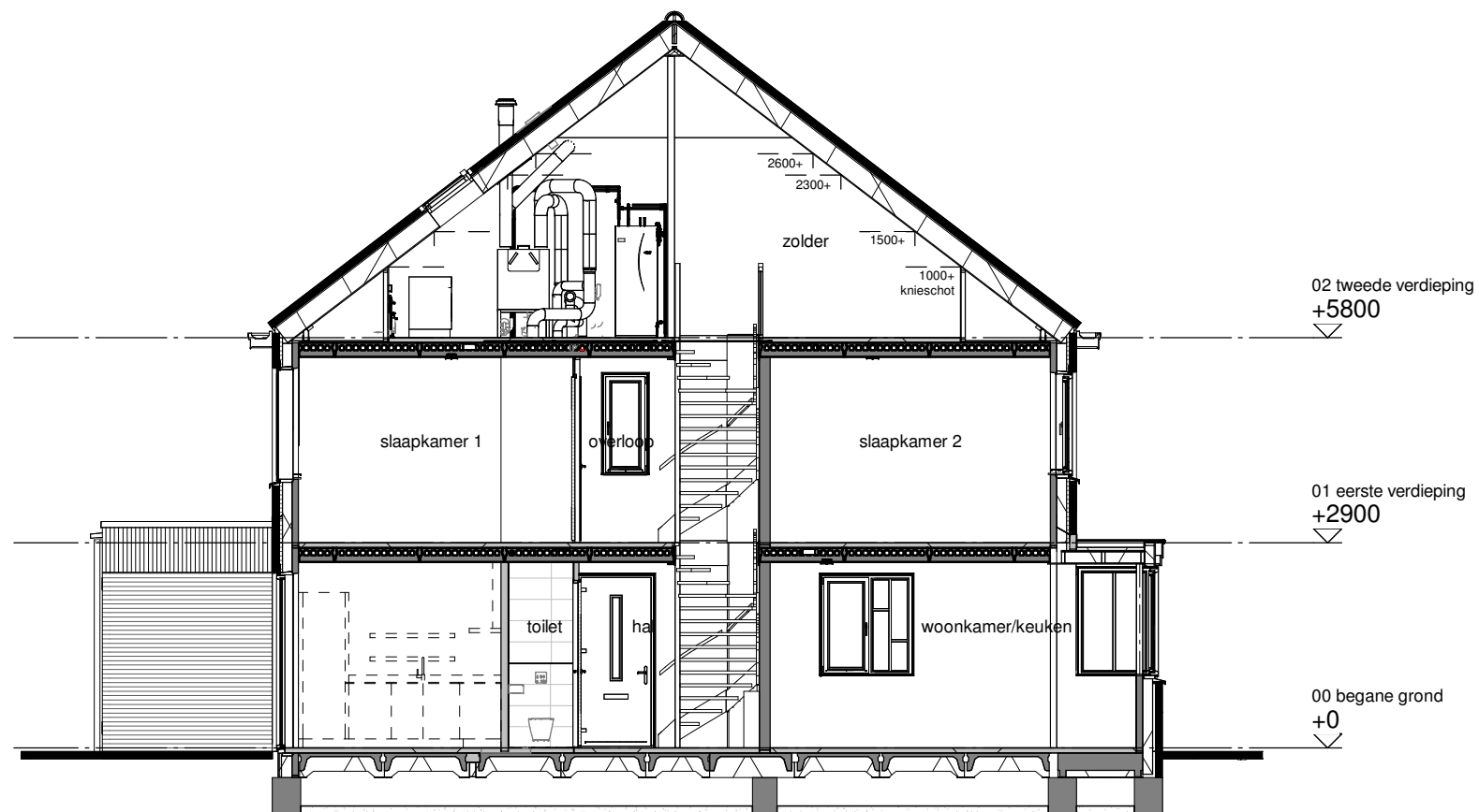
Doorsnede A
